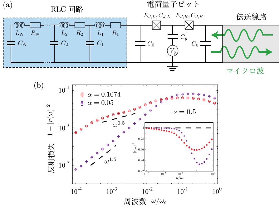
図 1. (a) スピン・ボソン模型で記述される超伝導回路と (b) s = 0.5 のマイクロ波反射損失 1 - |r(\omega)|^2 の計算結果。 \alpha は量子ビットと RLC 回路の間の結合強度。 \alpha が臨界値を取る場合、赤のプロットは臨界値より小さい値を取る場合をそれぞれ表している。
