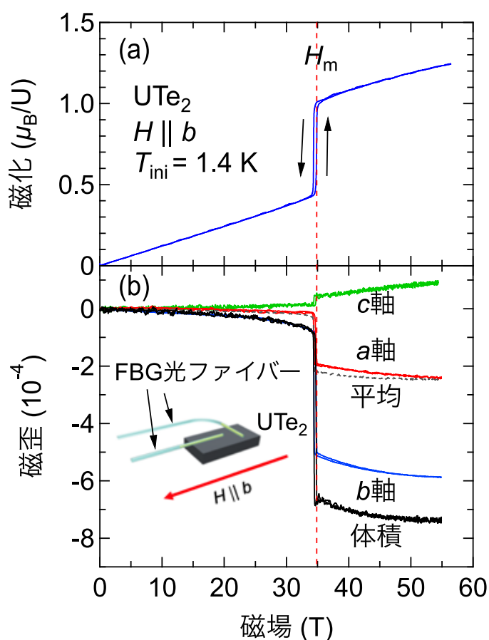
図 1. UTe_2 の b 軸に磁場( H )を印加したときの初期温度 1.4 K での(a)磁化と(b)各結晶軸方向の線磁歪と体積磁歪。内挿図は縦・横磁歪同時測定用セッティングの概念図。
